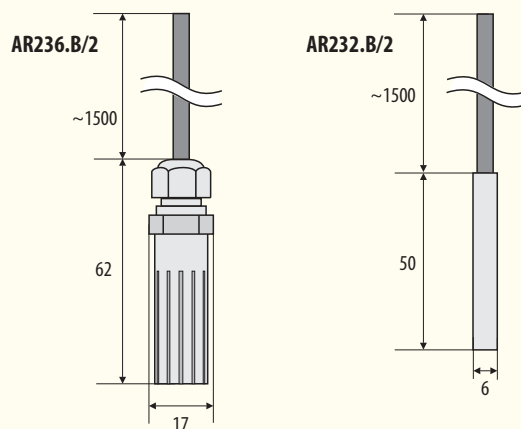
Wersja z sondą pomiarową na przewodzie
