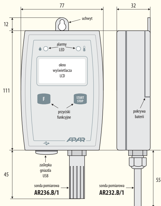
Wersja standard (sonda pomiarowa zintegrowana z obudową)
